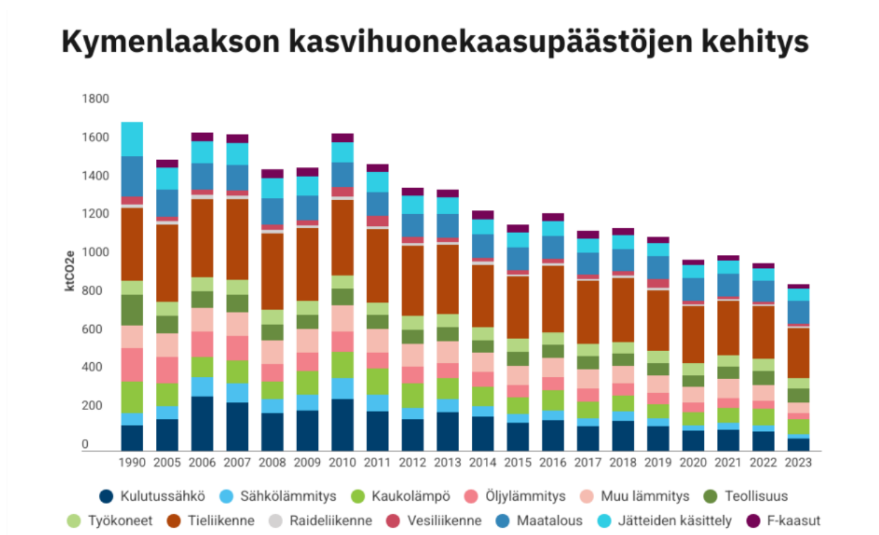
Kuva 5 Kymenlaakson Hinku-laskentasääntöjen mukaisten päästöjen kehitys vuosina 1990 ja 2005–2023. Lähde: Syke, hiilineutraalisuomi.fi
