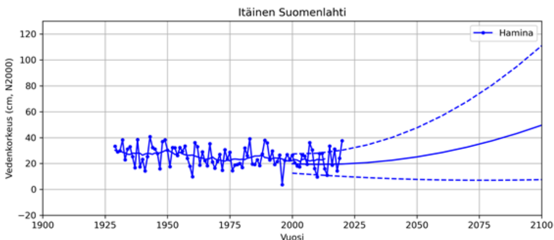
Kuva 4 Itäisen Suomenlahden mitattu merenpinnan nousu ja kolmen ilmastoskenaarion mukainen pysyvä merenpinnan nousu. Lähde: Suomen ilmastopaneeli 2021
