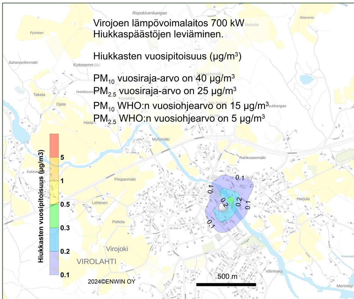
Kuva 5. Lämpölaitoksen päästöjen vaikutus hiukkasten vuosipitoisuuksiin Virojoella. Virolahdella tausta-asetalla v. 2023 \text{PM}_{2.5} vuosipitoisuus oli 3.6 \mu\text{g}/\text{m}^3 ja \text{PM}_{10} vuosipitoisuus 5 \mu\text{g}/\text{m}^3 .
